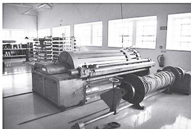
Urdideira e órgão com a teia
