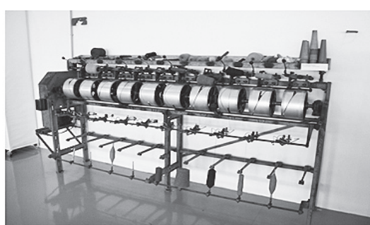
Bobinadeira Mecânica – J.M. Nicolau Raposo, Covilhã
