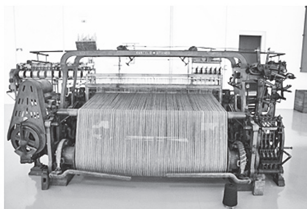
Tear C45 – Automecânica da Beira, Lda, Castelo Branco
